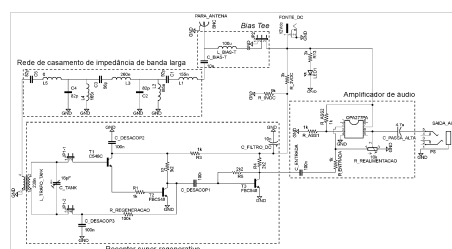
Fig. 2 – Circuito completo do receptor proposto. Nele, o sinal é tratado e amplificado para a saída de áudio.
