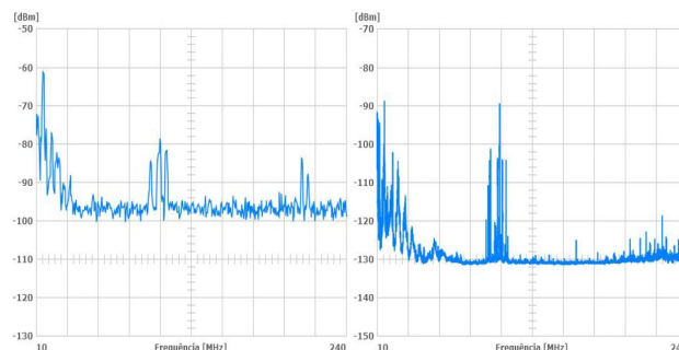
Fig. 3 – Característica do Espectro Eletromagnético na região do OES, na faixa de 10-240 MHz, em 2003 e 2009, respectivamente. Resultados que comprovam o potencial do OES para receber os arranjos interferométricos.
