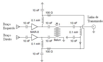
Fig. 1 – Diagrama representativo da estrutura da antena Fork e circuito completo da Antena Ativa do protótipo de rádio interferômetro do Observatório Espacial do Sul, em São Martinho da Serra.
